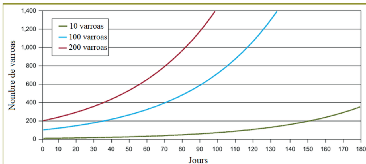
Figure 5 : Augmentation du taux d'infestation par Varroa sur 180 jours, en fonction du nombre initial de parasites dans la colonie. Seul un nombre faible de 10 varroas environ permet de rester sous le seuil critique de 1 000 varroas sur la période considérée. Issue de Managing varroa - The Food and Environment Research Agency (2015) .
